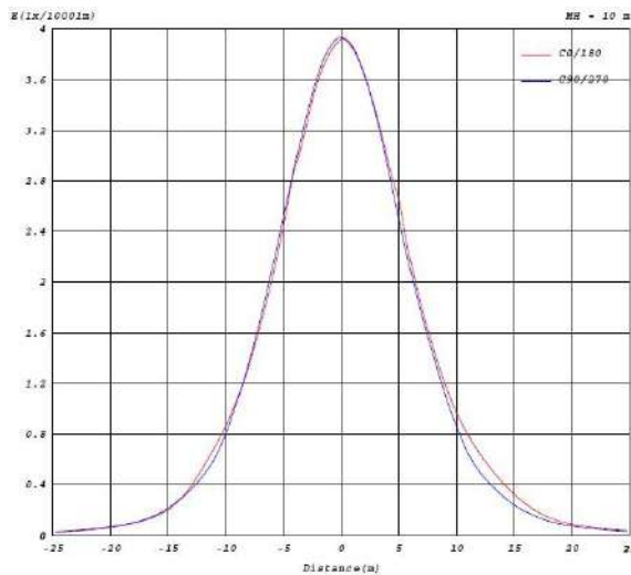
照度曲線
